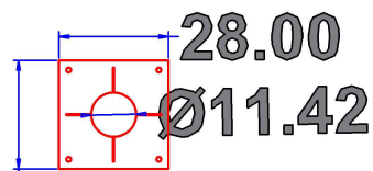
28.00 Ø11.42 PLANTA BAIXA FLANGE PARA BASE E CHUMBADOR MEDIDAS EM CM
